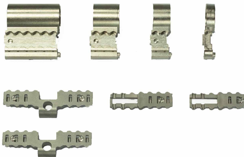
Slika: Sve duljine cilindra mogu se izvesti sa samo četiri različita dijela mosta i produžecima kućišta.
